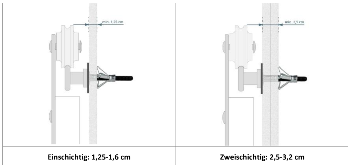
Gipskartonwand – Plattenlayout:
