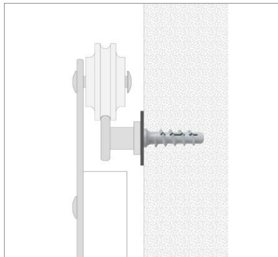
Porenbetonwand - layout:
